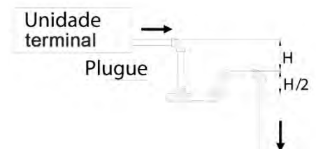
Figura 3-6.6: Armadilhas d'água na tubulação de drenagem
