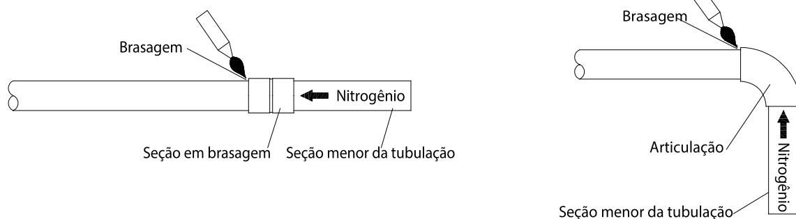
Figura 3-5.5: Fluxo do nitrogênio a partir do lado menor durante a soldagem
