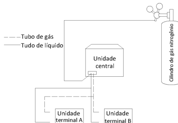
Figura 3-5.11: Lavagem de tubos usando nitrogênio
