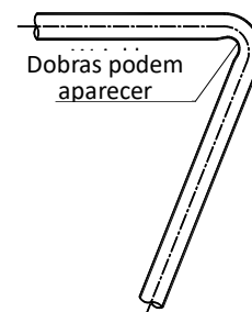
Figura 3-5.3: Arqueamento de tubos em mais de 90^\circ
