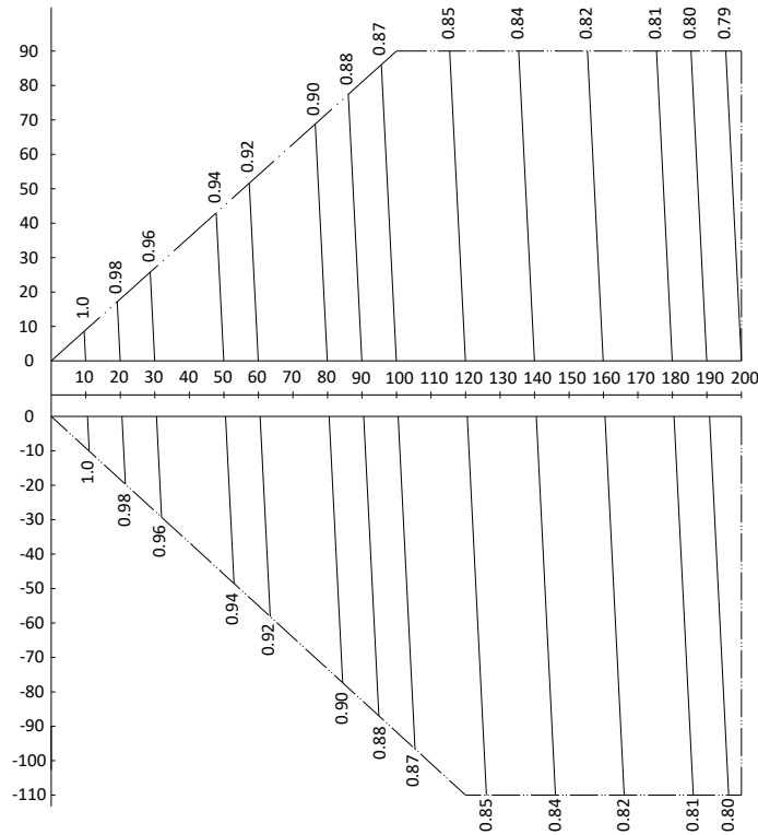
Figura 2-8.31: taxa de mudança na capacidade de resfriamento
