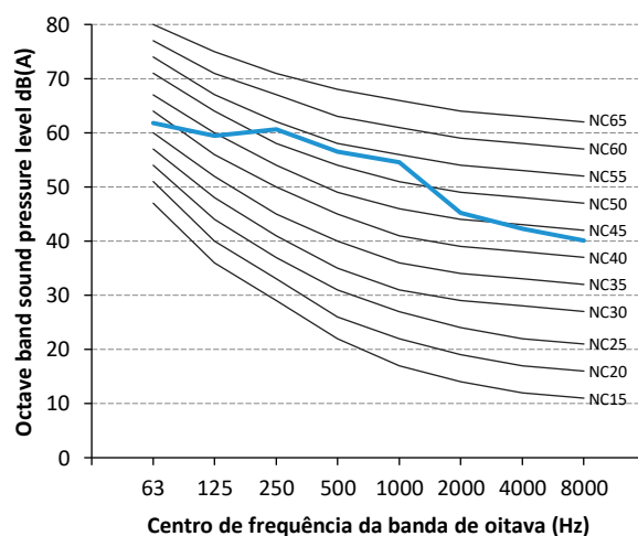
Figura 2-10.3 38VF010H119015 nível da banda de oitava
