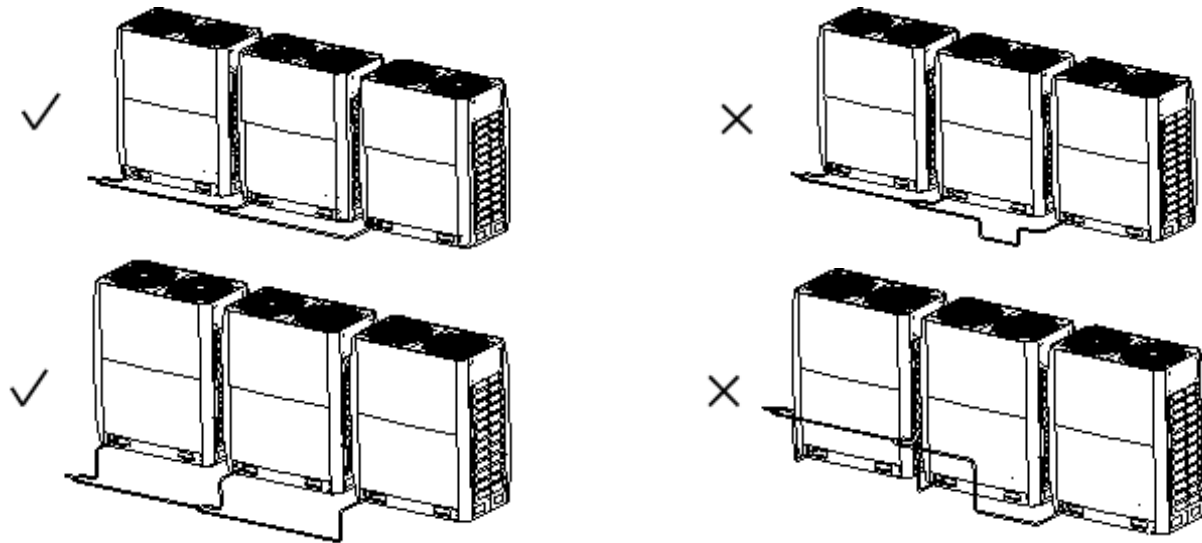
Figura 3-5.10: Conexões de tubulação entre as unidades centrais
