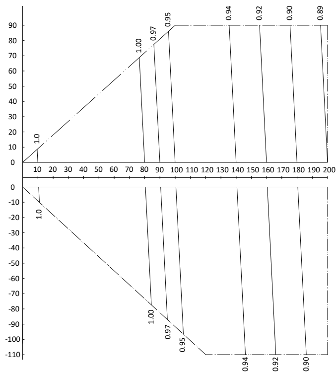
Figura 2-8.30: taxa de mudança na capacidade de aquecimento
