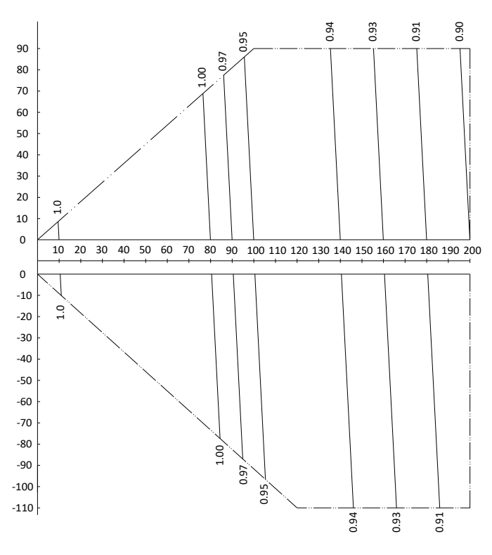
Figura 2-8.24: taxa de mudança na capacidade de aquecimento
