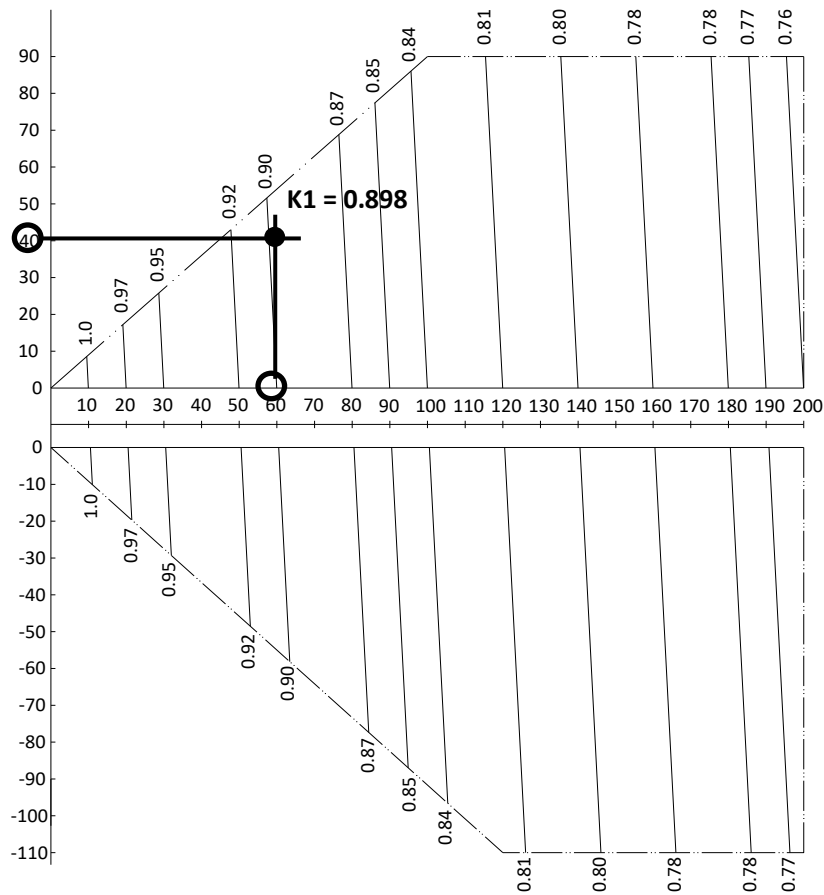
Figura 1-6.3: 38VF020H119015 taxa de mudança na capacidade de mudança
