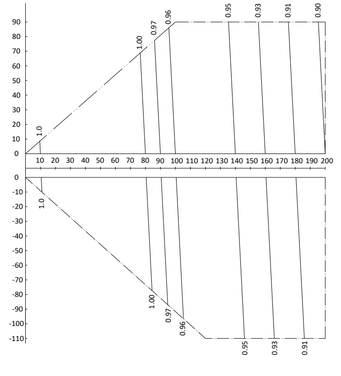
Figura 2-8.20: taxa de mudança na capacidade de aquecimento
