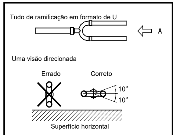
Figura 3-5.8: Orientação na articulação
