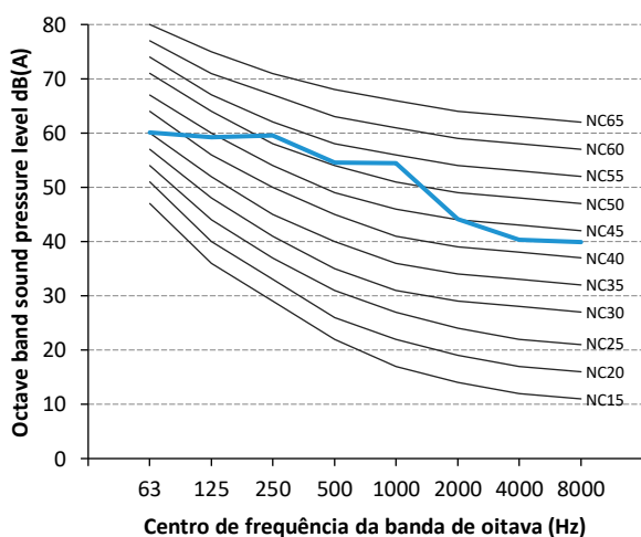
Figura 2-10.2 38VF008H119015 nível da banda de oitava
