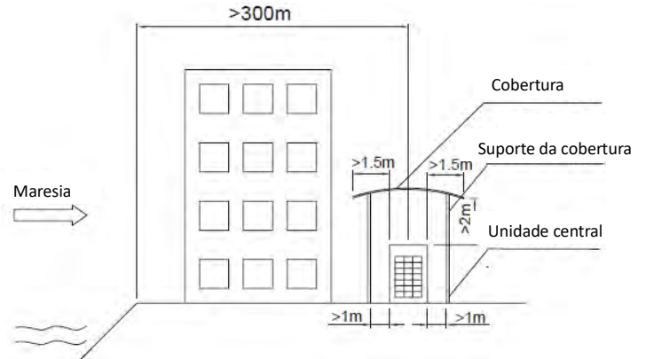
Figura 3-10.2: Instalação exterior sob uma cobertura
