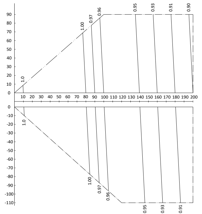
Figura 2-8.12: taxa de mudança na capacidade de aquecimento
